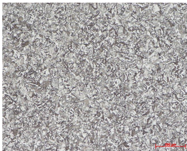
Aço Maraging VART300QA® após solubilização.
